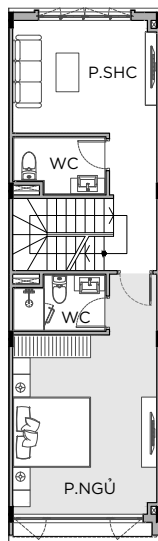
MẶT BẰNG TẦNG 2
