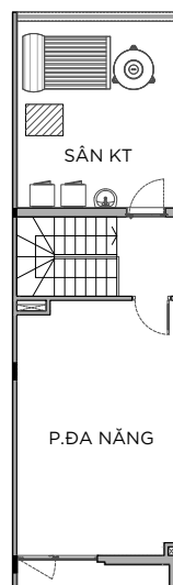
MẶT BẰNG TẦNG 5
