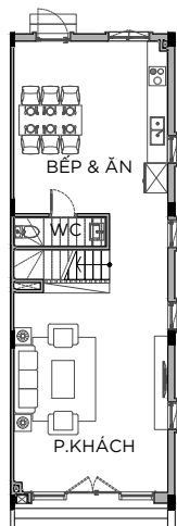
MẶT BẰNG TẦNG 1
