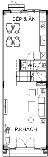
MẶT BẰNG TẦNG 1
