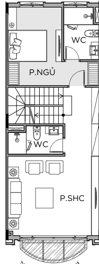
MẶT BẰNG TẦNG 2
