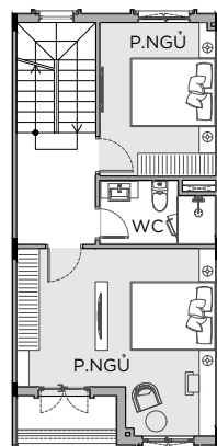
MẶT BẰNG TẦNG 4
