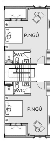
MẶT BẰNG TẦNG 3
