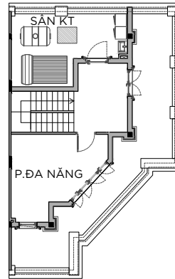
MẶT BẰNG TẦNG 5
