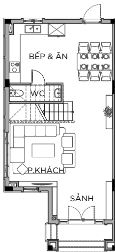
MẶT BẰNG TẦNG 1
