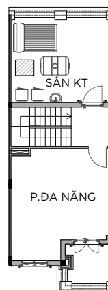
MẶT BẰNG TẦNG 5
