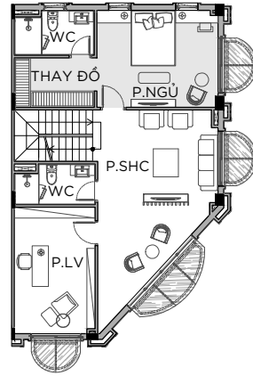
MẶT BẰNG TẦNG 2
