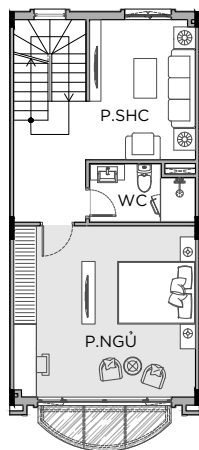
MẶT BẰNG TẦNG 2
