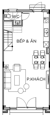
MẶT BẰNG TẦNG 1
