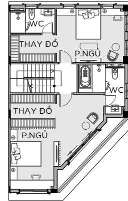
MẶT BẰNG TẦNG 3
