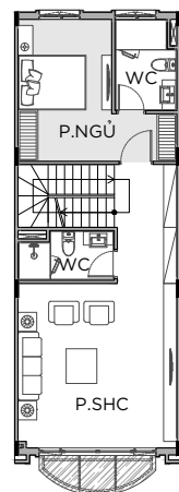
MẶT BẰNG TẦNG 2
