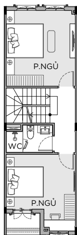
MẶT BẰNG TẦNG 4
