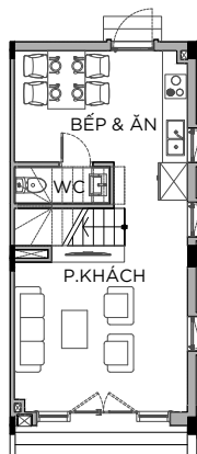
MẶT BẰNG TẦNG 1
