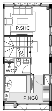
MẶT BẰNG TẦNG 2
