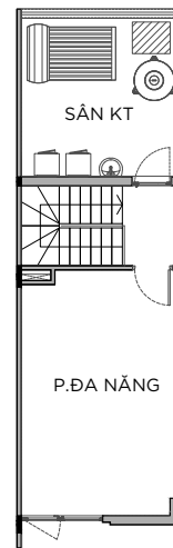
MẶT BẰNG TẦNG 5
