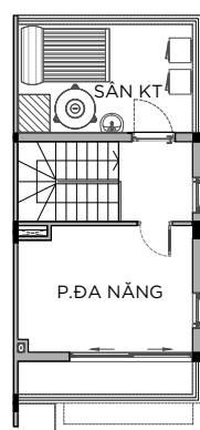
MẶT BẰNG TẦNG 5
