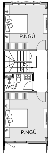
MẶT BẰNG TẦNG 4
