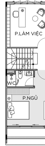
MẶT BẰNG TẦNG 3
